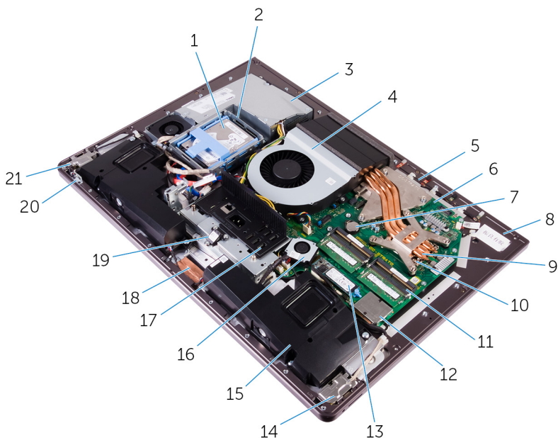
Figure 2 : Vue interne de l'ordinateur (écran non tactile)
